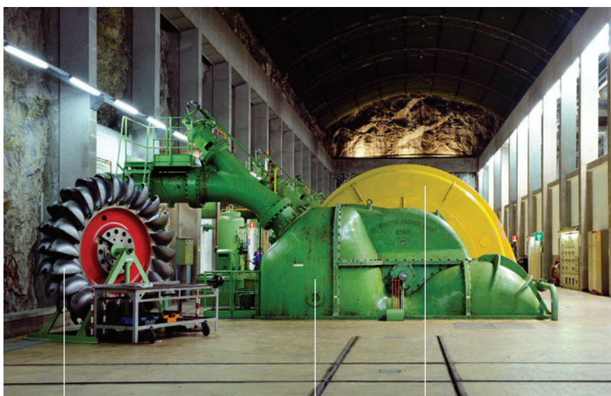
Girante Pelton
